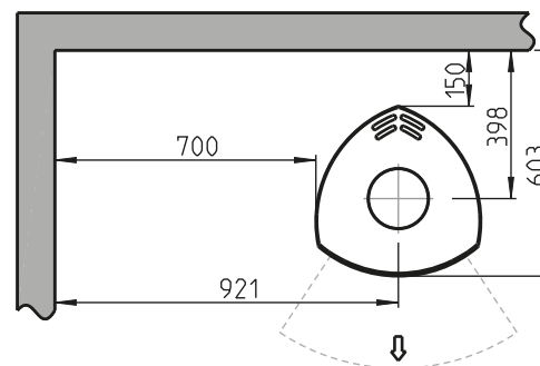
Minimale afstand tot brandbare muur
