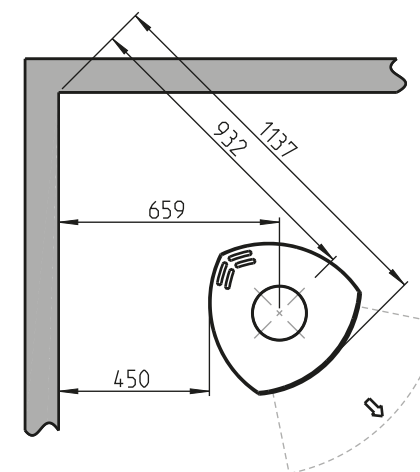
Minimale afstand tot brandbare muur
