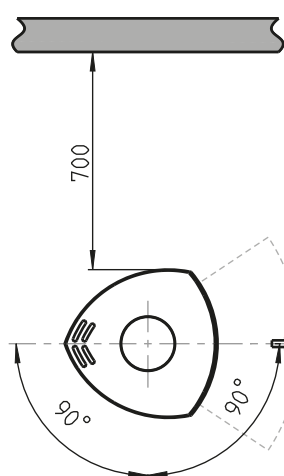
Afstand tot brandbare muur met draaibaar voetstuk
