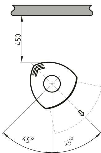
Afstand tot brandbare muur met draaibaar voetstuk
