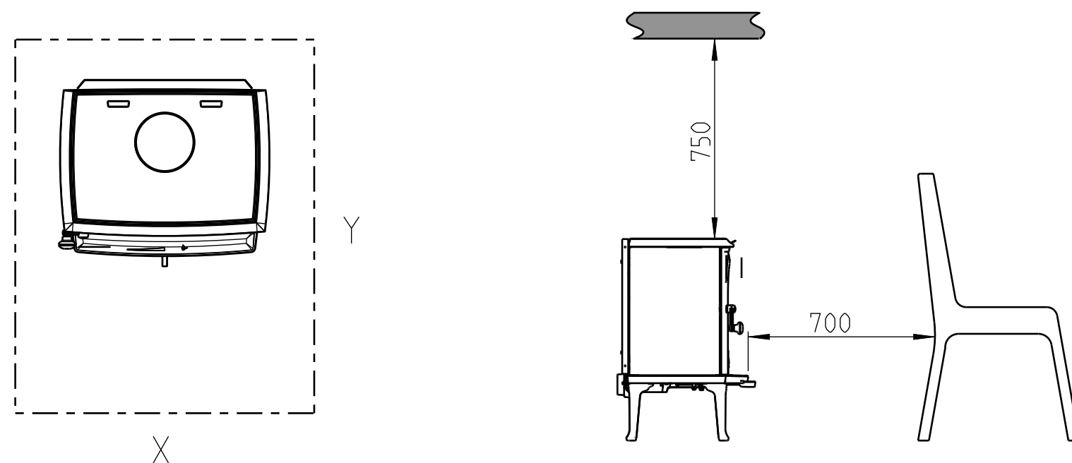
Minimale afstand tot plafond
